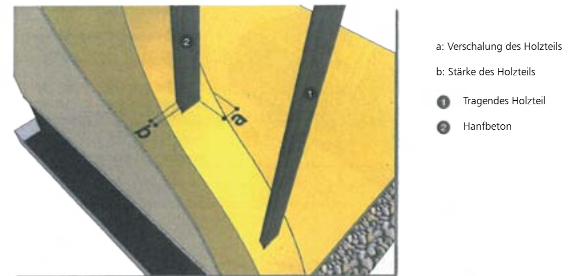
Abb. 9: Mindestdicke der Verschalung (a) je nach Stärke (b) der tragenden Holzteile
